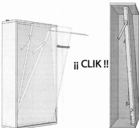
11. Escucharemos un "CLICK" que nos indica que los pistones se han activado correctamente.
